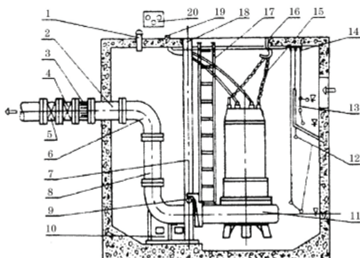
Рис. 8 Стационарная установка
